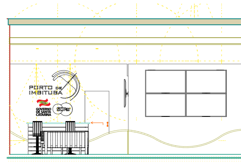
Elevação 3
